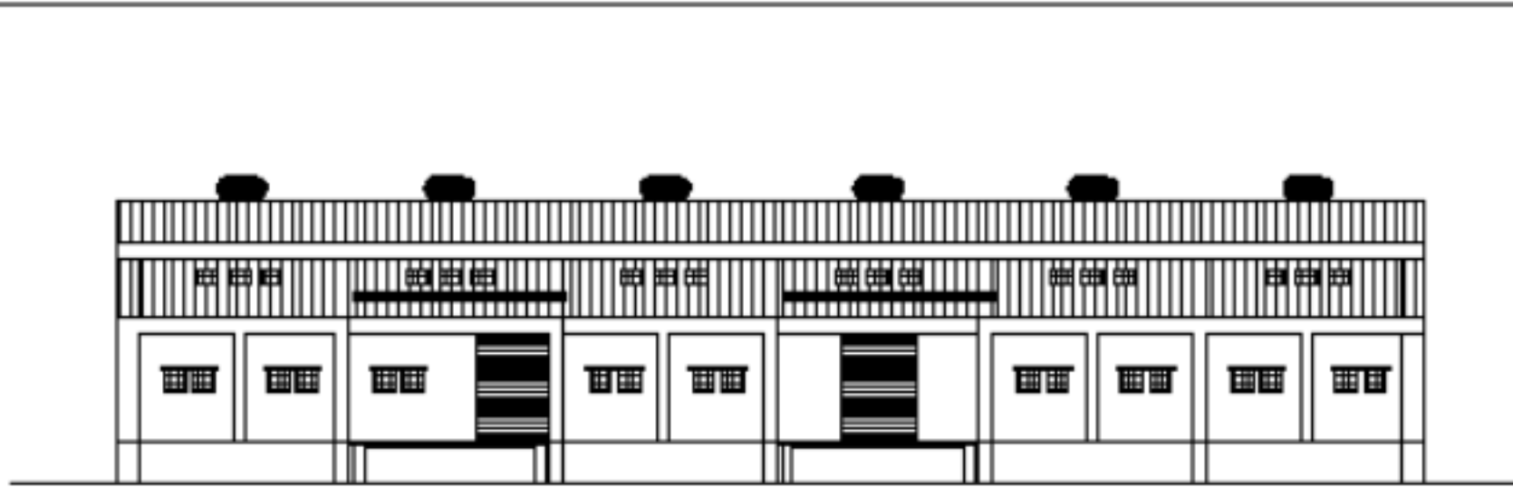
ELEVATION
